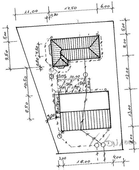
Auszug Lageplan
